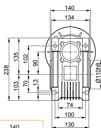
Albero uscita / Output shaft
