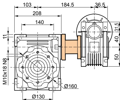
Albero uscita / Output shaft
