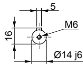
Albero entrata / Input shaft
