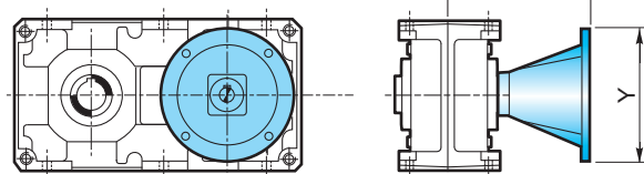
ZF..B
