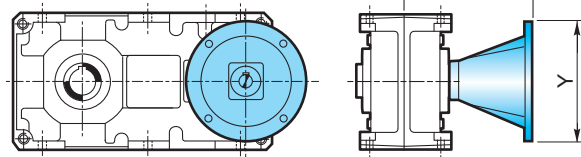
ZF..C
