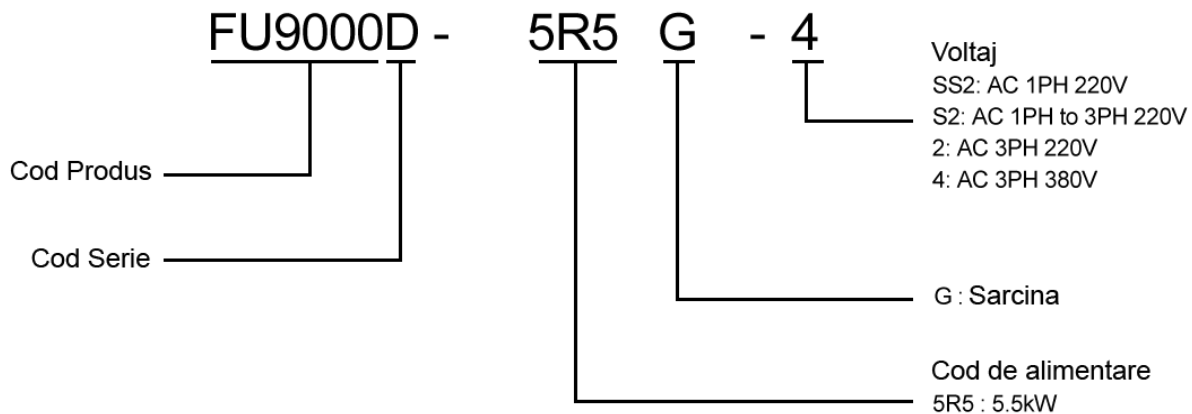
Figura 1-1 Reguli de denumire si placuta de identificare a FU9000D
